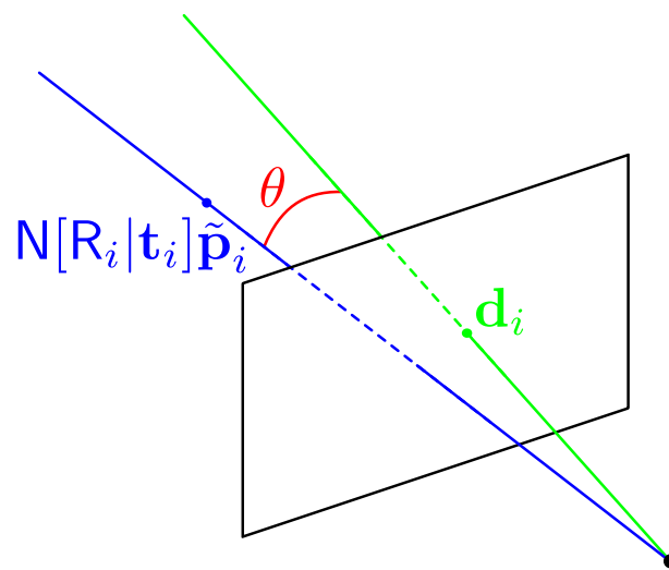
FIGURE V.1 – Minimiser l'erreur algébrique revient à minimiser le produit vectoriel \left[ \tilde{d}_i \right]_{\wedge} N[R_i | t_i] \tilde{p}_i . Sa norme est ainsi minimisée et comme d_i et N[R_i | t_i] \tilde{p}_i sont des vecteurs non-nuls, nous minimisons donc l'angle \theta entre eux. Ces deux vecteurs sont donc rapprochés l'un de l'autre jusqu'à être éventuellement colinéaires.
